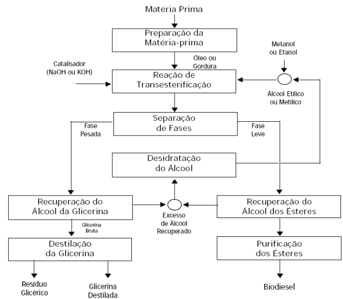
Fluxograma do Processo de Produção de Biodiesel
